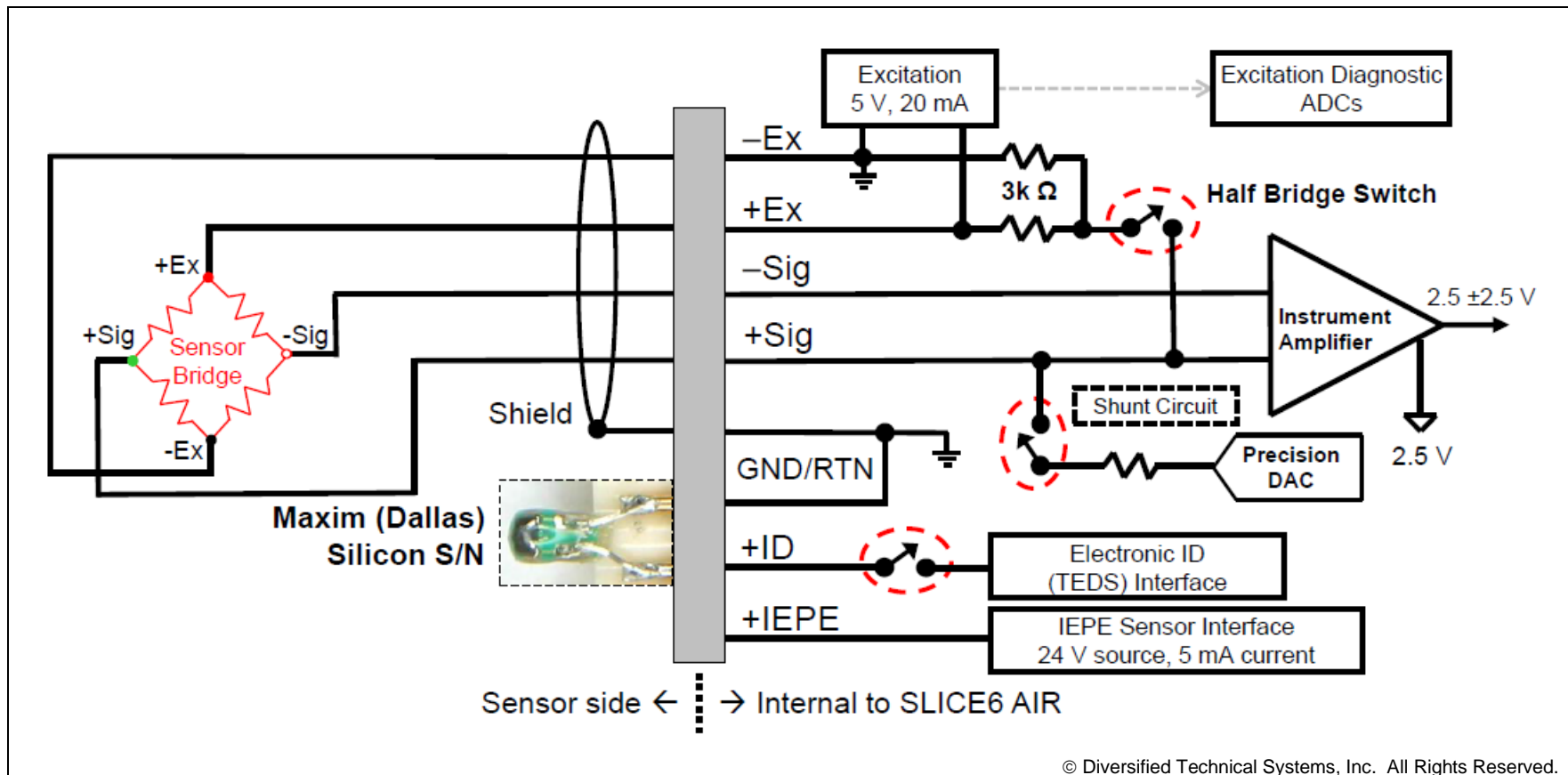
SLICE6 AIR DAS Sensor Interface
